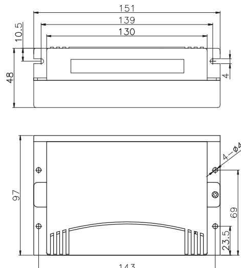
(d) Mechanical specifications of the EM806
